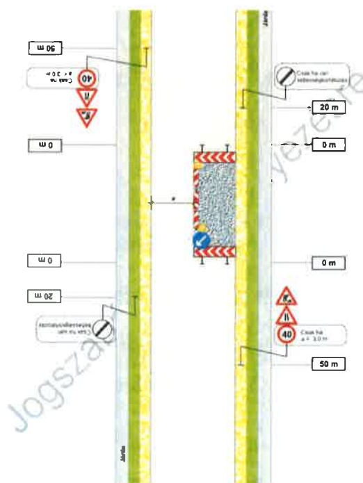
12. ábra – Egy forgalmi sáv lezárása két forgalmú úton (forgalomirányítás nélkül)
